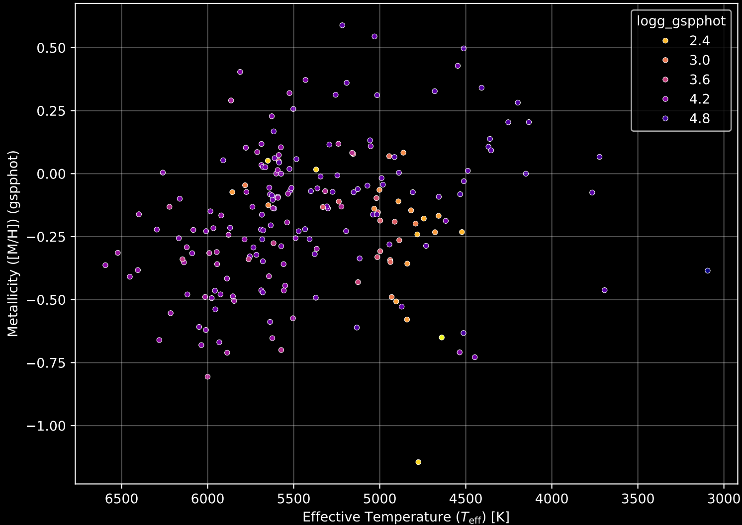
APOGEE DR17 Field: [110+66_MGA] Stellar Population Parameters (n= 204)
